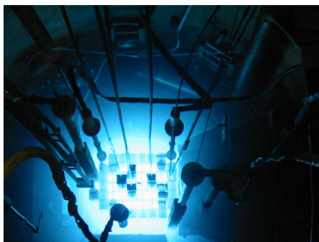
Fotografia rdzenia reaktora MARIA – źródło IEA.
